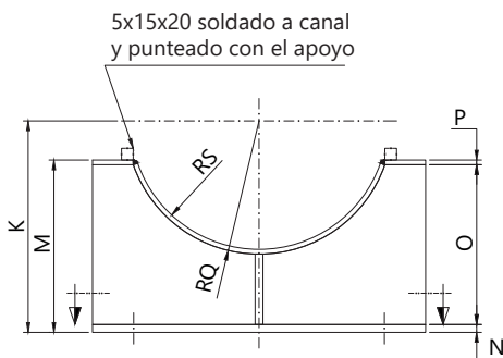
Alzado del soporte de media luna
