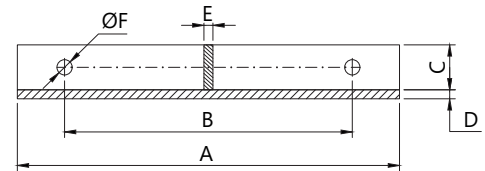
Planta del soporte de media luna
